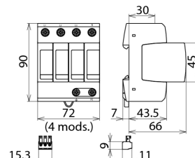
Målskitse DG M TT 275 FM
